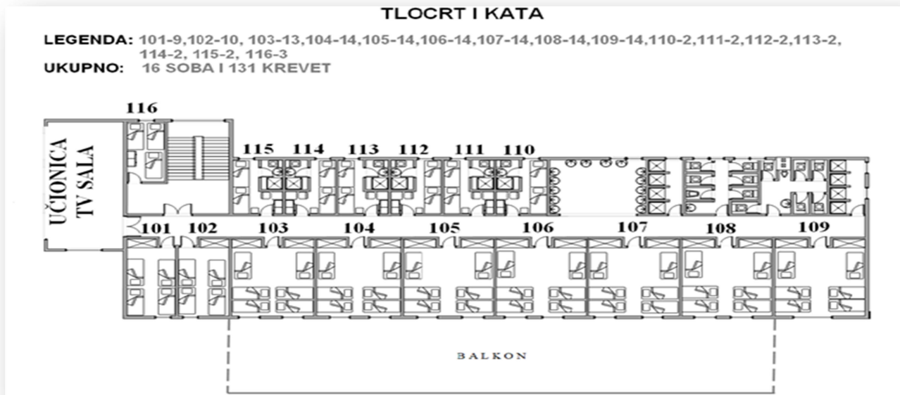
Slika 2: Tlocrt I. kata
